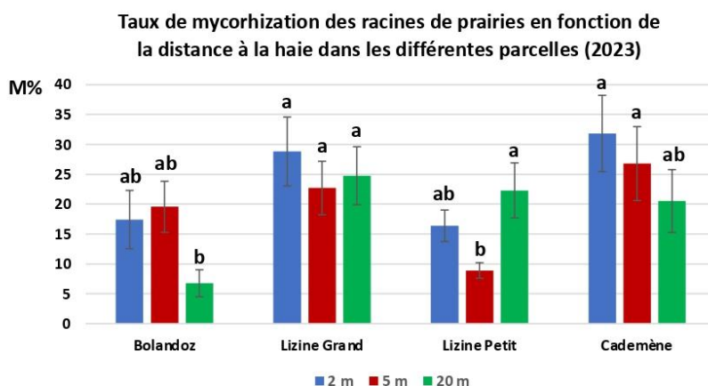
Figure 1. Moyenne des taux de mycorhization (M%) des racines prélevées le 6 juin 2023 au niveau des parcelles de Bolandoz, Lizine Grand, Lizine Petit et Cademène à 2, 5 et 20 mètres de la haie (moyenne \pm erreur standard de la moyenne ; test de Kruskal-Wallis, P < 0,05 ).
