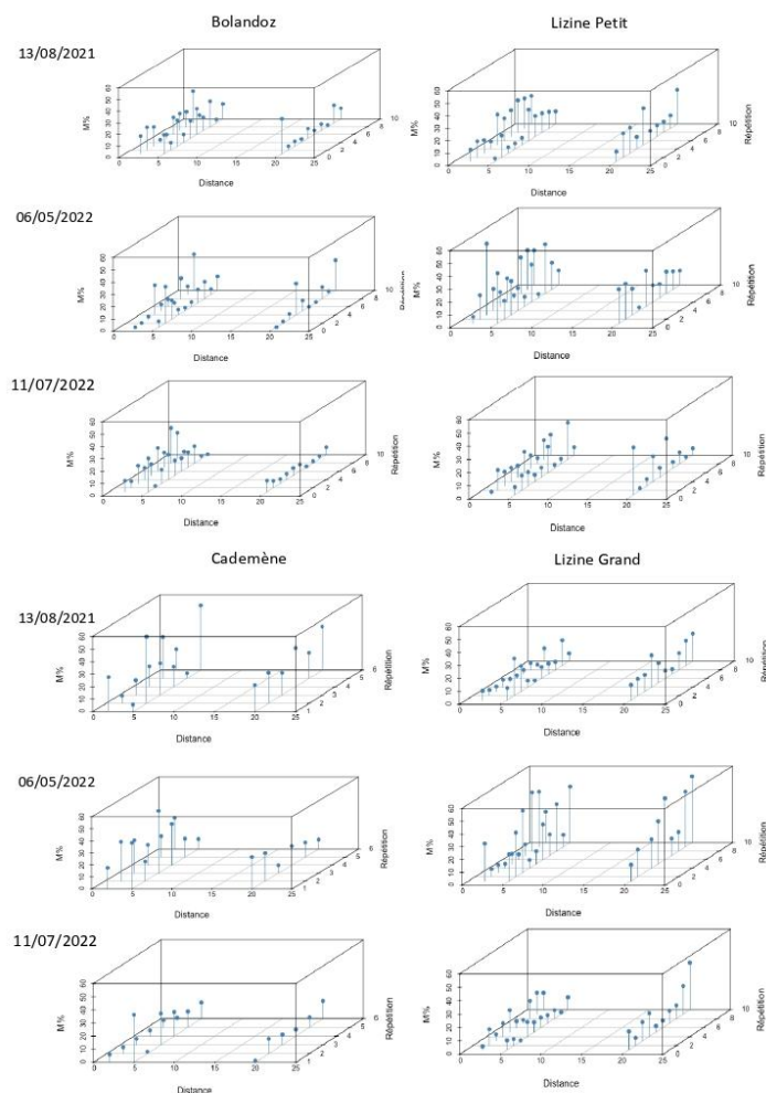
Figure 2. Taux de mycorhization des différents échantillons de racines dans les parcelles de Bolandoz, Cademène, Lizine Grand et Lizine Petit, à 2 m, 5 m et 20 m de la haie et à chaque date de prélèvement.
