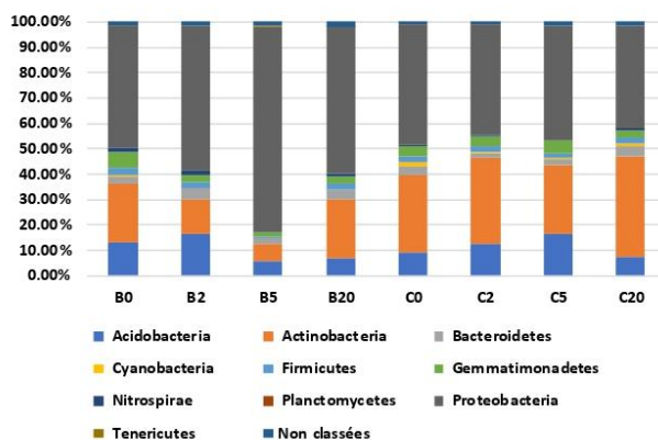
Figure 3. Abondance relative des phyla de bactéries dans le sol des parcelles de Bolandoz (B) et Cademène (C) à 0, 2, 5 et 20 mètres de la haie.
