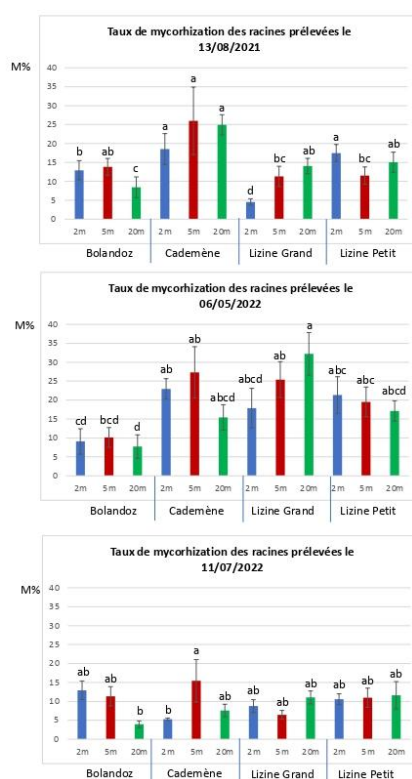
Figure 3. Taux de mycorhization (M%) des racines prélevées en 2021 et 2022 au niveau des parcelles de Bolandoz, Cademène, Lizine Grand et Lizine Petit en fonction des distances à la haie (moyenne \pm erreur standard de la moyenne)
