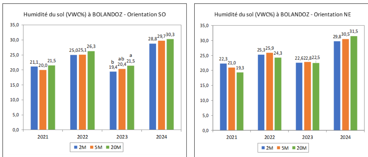
Figure 92 : évolution annuelle de l'humidité du sol selon la distance et l'orientation de la haie.
