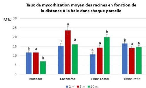
Figure 4. Taux de mycorhization (M%) moyen des racines prélevées en 2021 et 2022 au niveau des parcelles de Bolandoz, Cademène, Lizine Grand et Lizine Petit en fonction des distances à la haie (moyenne \pm erreur standard de la moyenne).
