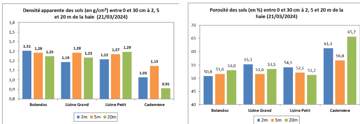
Figure 72 : densité apparente et porosité des sols par site d'étude et par distance à la haie en 2024.
