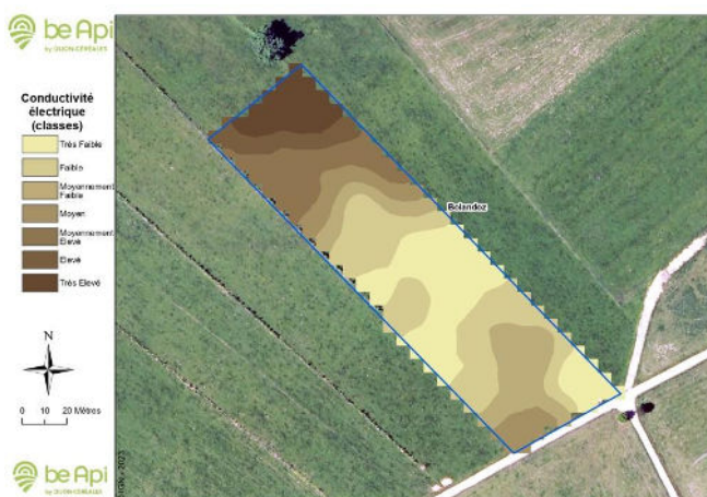
Figure 28 : carte de la conductivité à Bolandoz.
