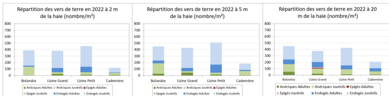
Figure 101 : répartition des effectifs de vers de terre en 2022 à 2 m (gauche), 5 m (milieu) et 20 m (droite) des haies 4 sites suivis.
