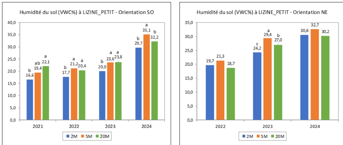
Figure 96 : évolution annuelle de l'humidité du sol à Lizine Petit selon la distance et l'orientation de la haie.
